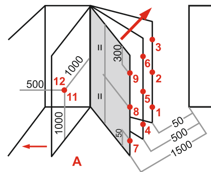
Basculante Tilting doors Basculantes Kipptore Porte Basculante
