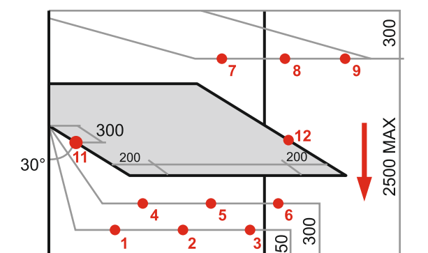
Basculante Tilting doors Basculantes Kipptore Porte Basculante
