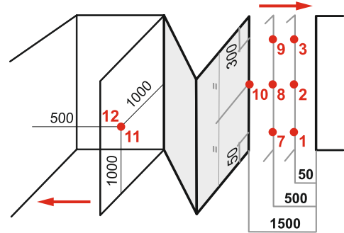
Cancello battente (singola e doppia anta) Swing gate (single and double leaf) Cancelas batientes (de una y dos hojas) Drehtor (Einzel- und Doppelblatt) Portail à battant (à un ou deux vantaux)
